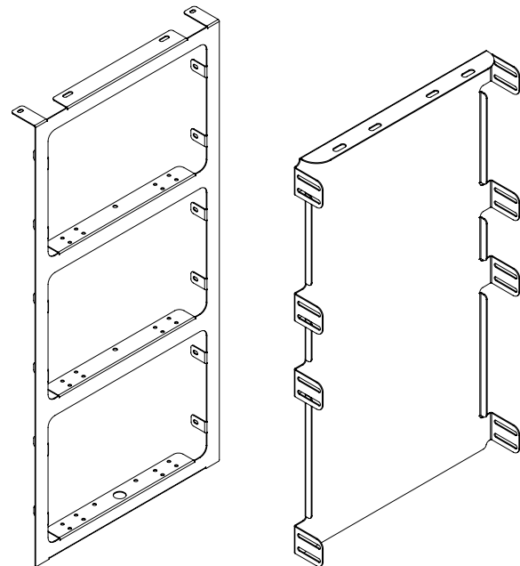
35.1 – 1x
